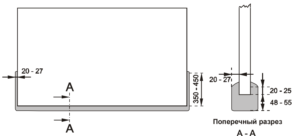
Рис. 7 Обивка щита
