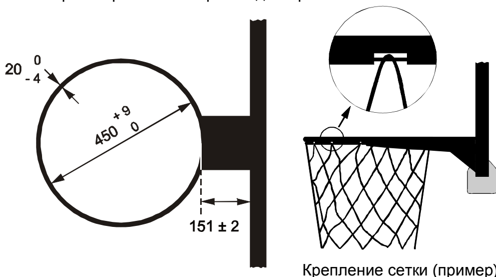
Рис. 4 Кольцо
