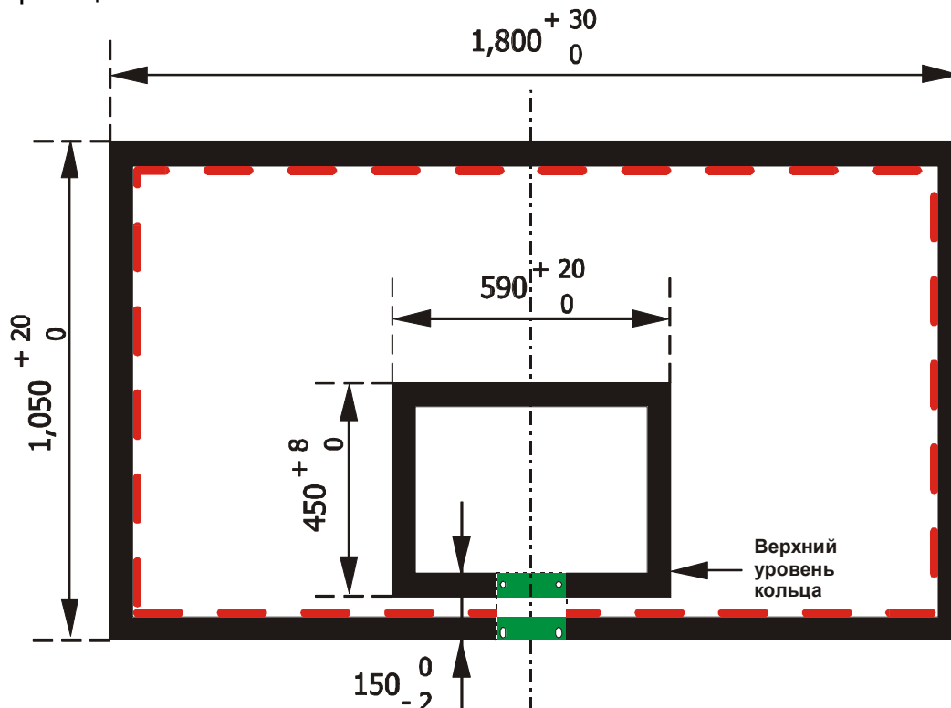
Рис. 2 Разметка щита
