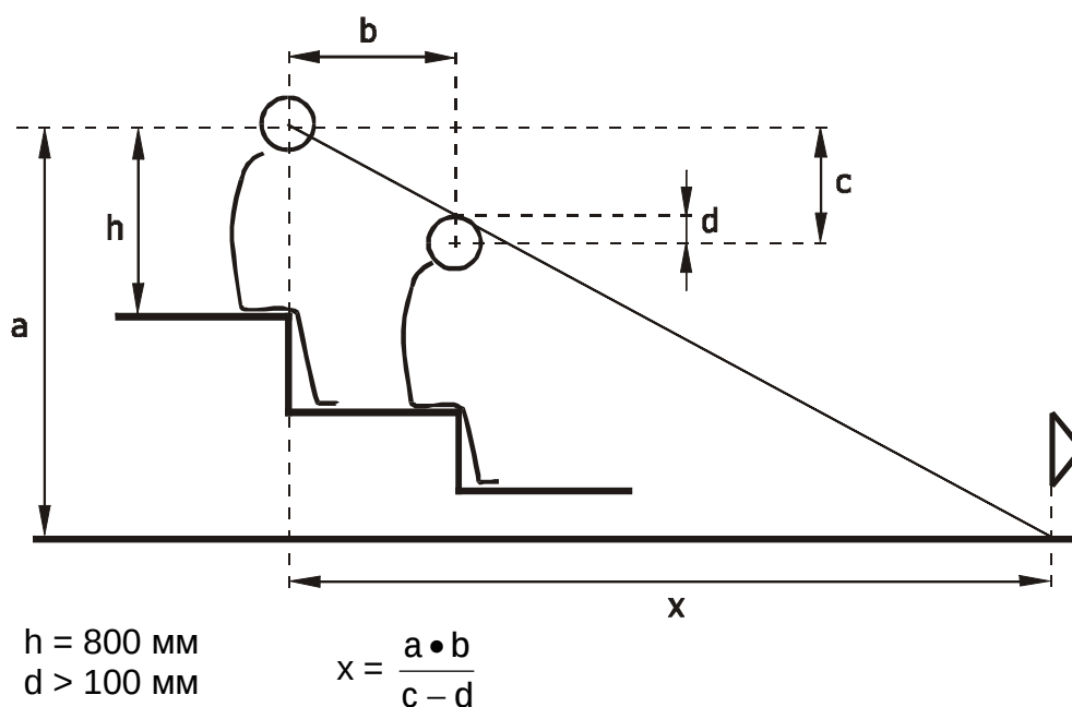
Рис. 13 Линия видимости зрителей
